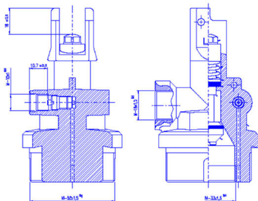
DETALLE PLANO VÁLVULA EXTINTOR PP50P
